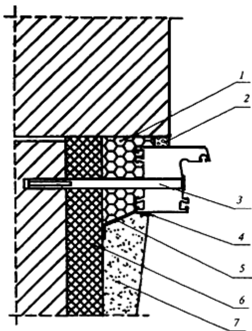
Рисунок А.1 - Узел бокового примыкания оконного блока к проему с четвертью в стене из кирпича, с отделкой внутреннего откоса штукатурным раствором
