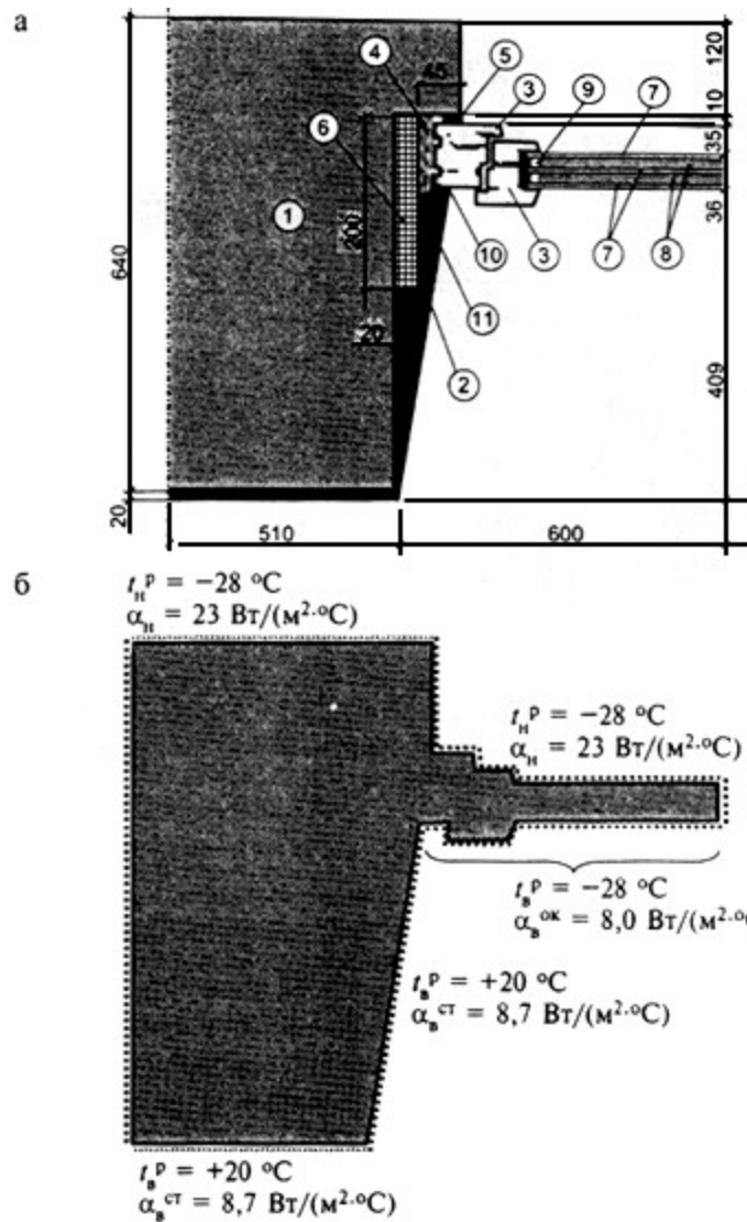
Рисунок Г.2 - Расчетная схема (а) и схема задания граничных условий (б) узла примыкания оконного блока к оконному проему
