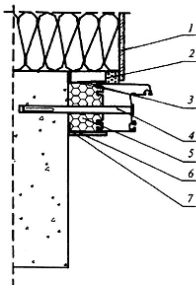
Рисунок А.8 - Узел бокового примыкания оконного блока к проему стены из бетона с наружным утеплением фасада и установкой внутреннего декоративного нащельника
