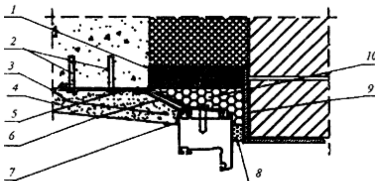
Рисунок А.5 - Узел верхнего примыкания оконного блока к перемычке из стального уголка в проеме многослойной стены с облицовкой кирпичом
