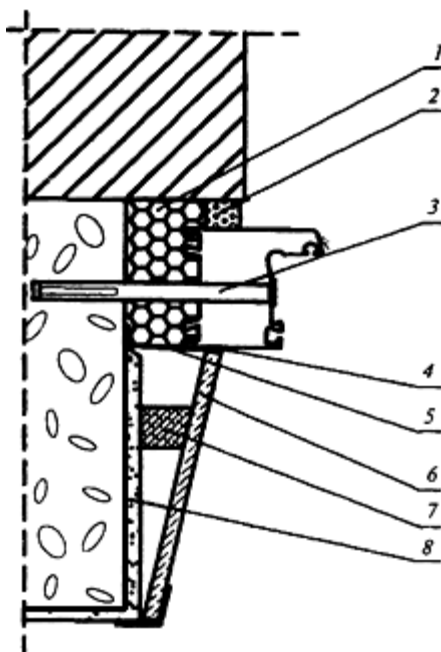
Рисунок А.6 - Узел бокового примыкания оконного блока к проему с четвертью в стене из ячеистобетонных блоков (плотностью 400-450 \text{ кг/м}^3 ) с облицовкой кирпичом и отделкой внутреннего откоса панелью
