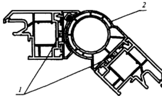
Рисунок А.16 - Узел углового соединения оконных коробок
