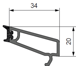
Штапик для стекла 4 мм Арт. 5804
