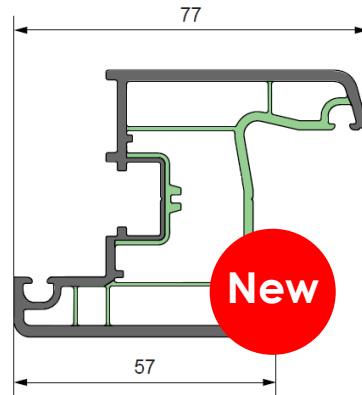
Створка (коэкс) Арт. 5802K
