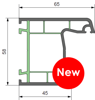
Рама (коэкс) Арт. 5801K
