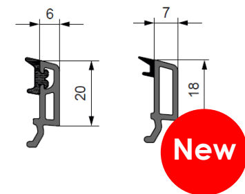
Штапики для стеклопакета 32 мм Арт. 5832 Арт. 5832-1
