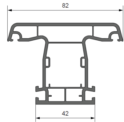
Импост Арт. 5803
