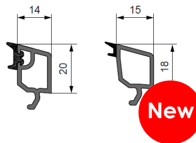
Штапики для стеклопакета 24 мм Арт. 5824 Арт. 5824-1
