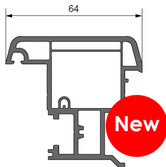
Штульп Арт. 5813
