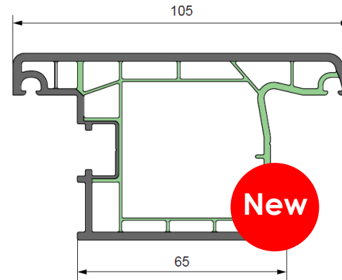
Т-створка дверная (коэкс) Арт. 5812K
