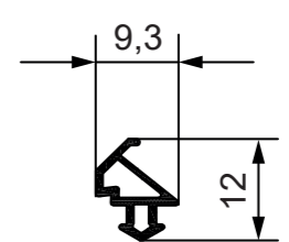
Уплотнитель притвора Арт. DF-228 Арт. DF-228G (серый)
