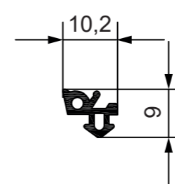
Уплотнитель стеклопакета Арт. DG-120 Арт. DG-120G (серый)
